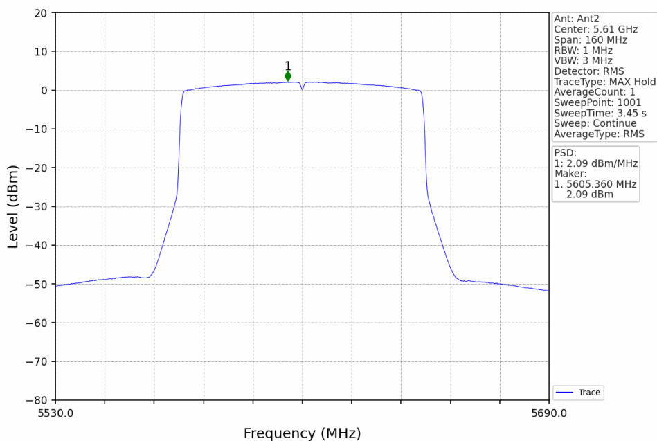
802.11ax(HEW80)_HCH_5610MHz_RU996_Left_MIMO_NTNV
