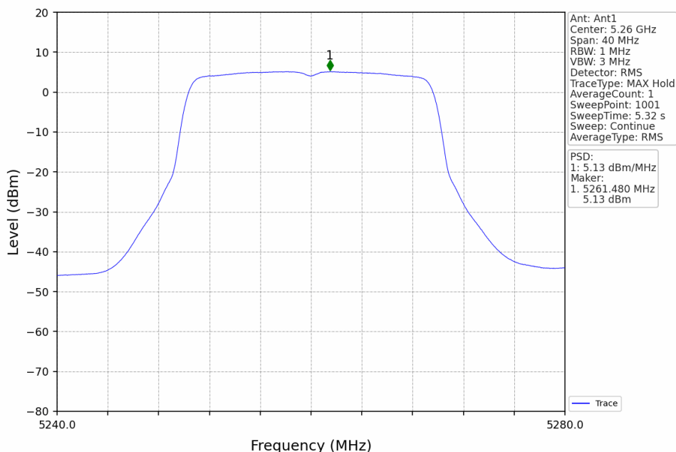
802.11ax(HEW20)_LCH_5260MHz_RU242_Left_Ant1_NTNV
