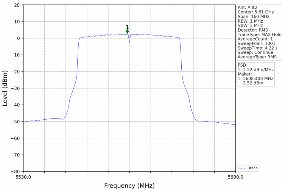
802.11ac(VHT80)_HCH_5610MHz_MIMO_NTNV
