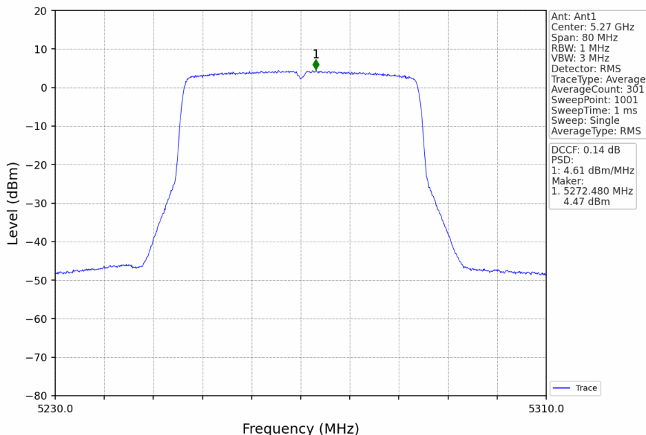
802.11ax(HEW40)_LCH_5270MHz_RU484_Left_Ant1_NTNV
