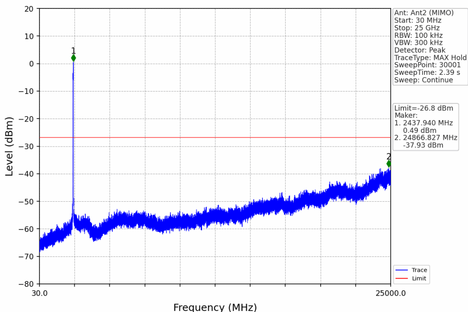
802.11ax(HEW40)_LCH_2422MHz_RU484_Left_Ant2 (MIMO)_NTNV
