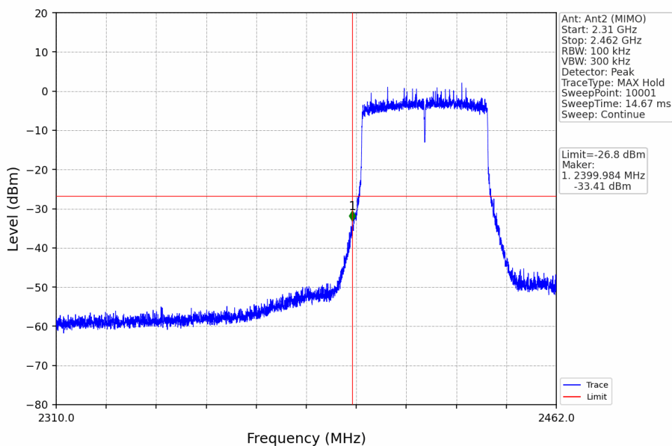
802.11ax(HEW40)_LCH_2422MHz_RU484_Left_Ant2 (MIMO)_NTNV
