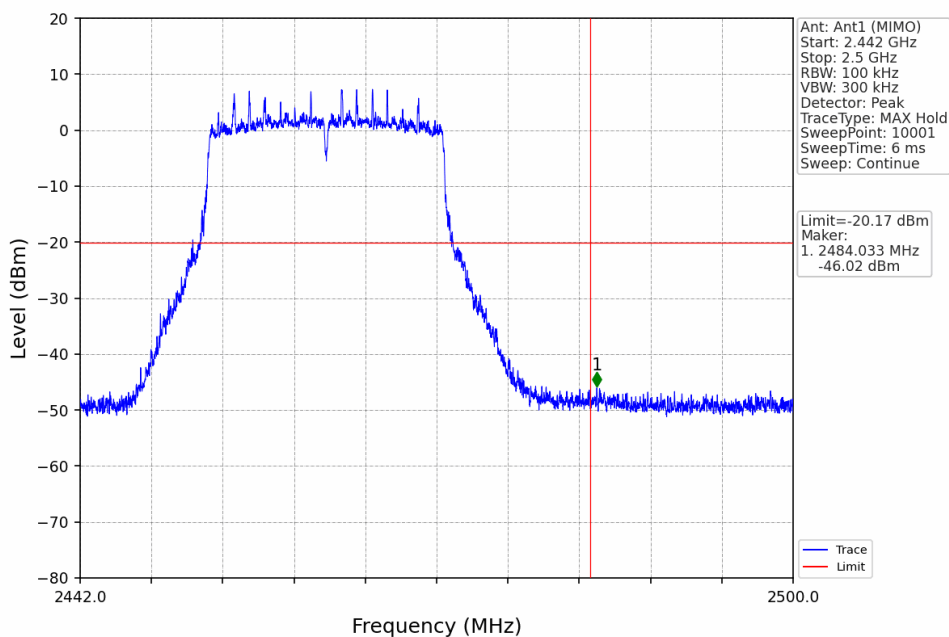
802.11ax(HEW20)_HCH_2462MHz_RU242_Left_Ant1 (MIMO)_NTNV
