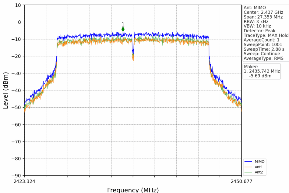
802.11ax(HEW20)_MCH_2437MHz_RU242_Left_MIMO_NTNV
