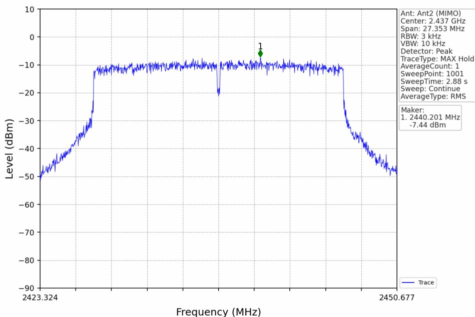
802.11ax(HEW20)_MCH_2437MHz_RU242_Left_MIMO_NTNV
