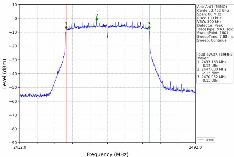
802.11ax(HEW40)_HCH_2452MHz_RU484_Left_Ant1 (MIMO)_NTNV
