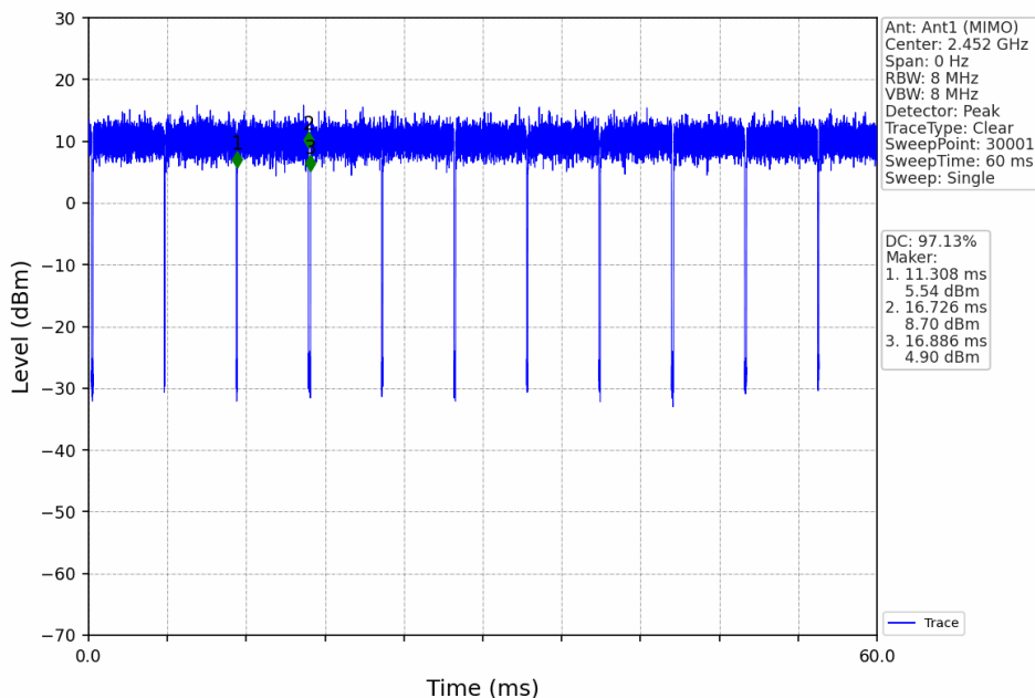
802.11ax(HEW40)_HCH_2452MHz_RU484_Left_Ant1 (MIMO)_NTNV
