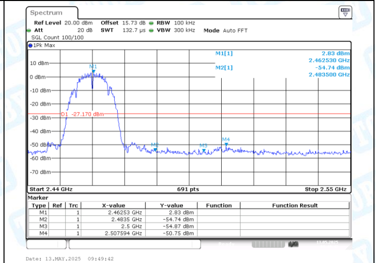
11B-CDD-Ant2-2462-PASS
