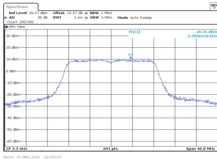
11A-MIMO_Ant1_5200
