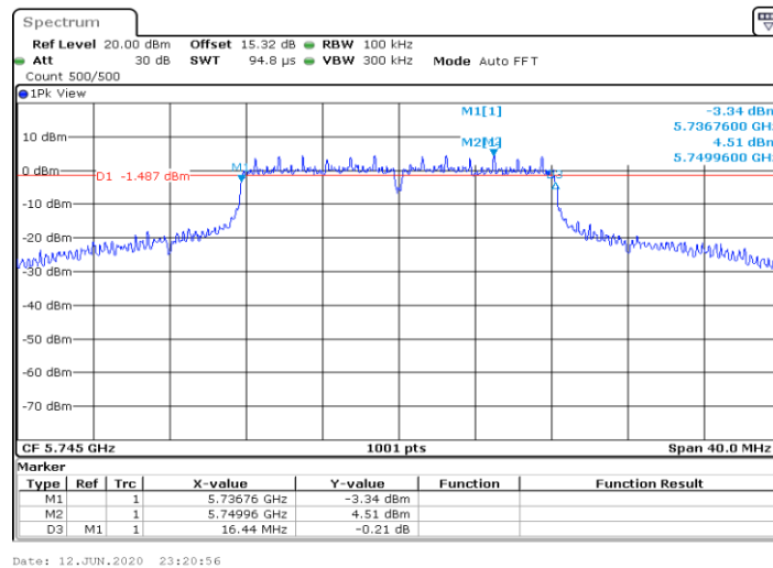
11A-MIMO_Ant2_5745
