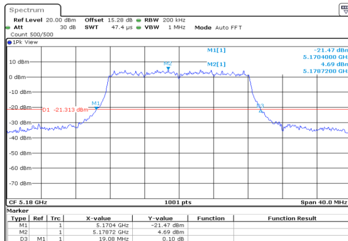
11A-MIMO_Ant2_5180
