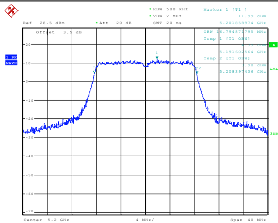
11A-MIMO_Ant1_5200
