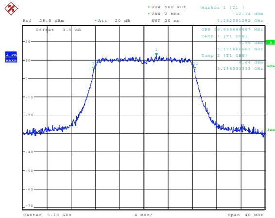
11A-MIMO_Ant2_5180
