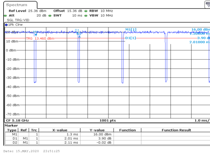
11A-MIMO_Ant2_5180
