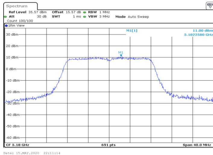
11A-MIMO_Ant2_5180
