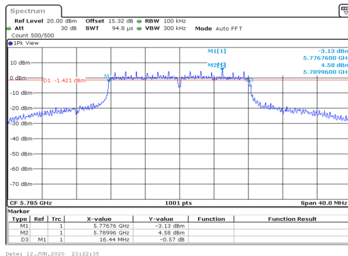
11A-MIMO_Ant1_5785
