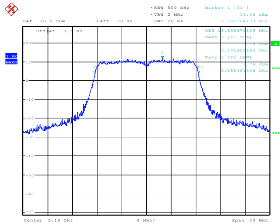
11A-MIMO_Ant1_5180
