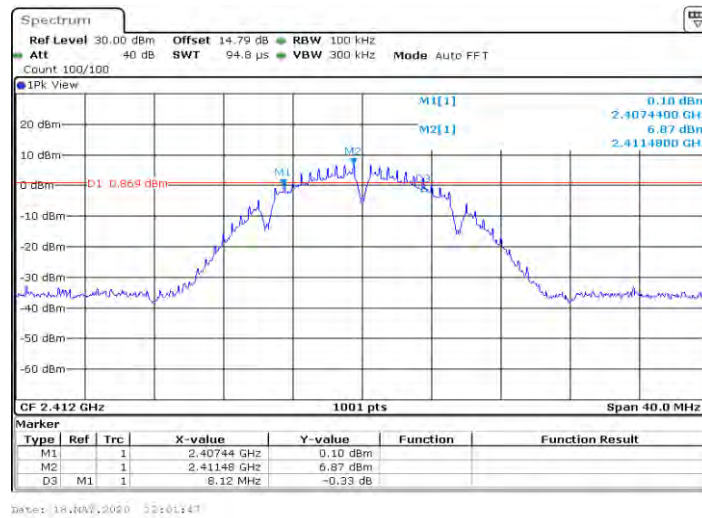
11bMIMO_Ant2_2412
