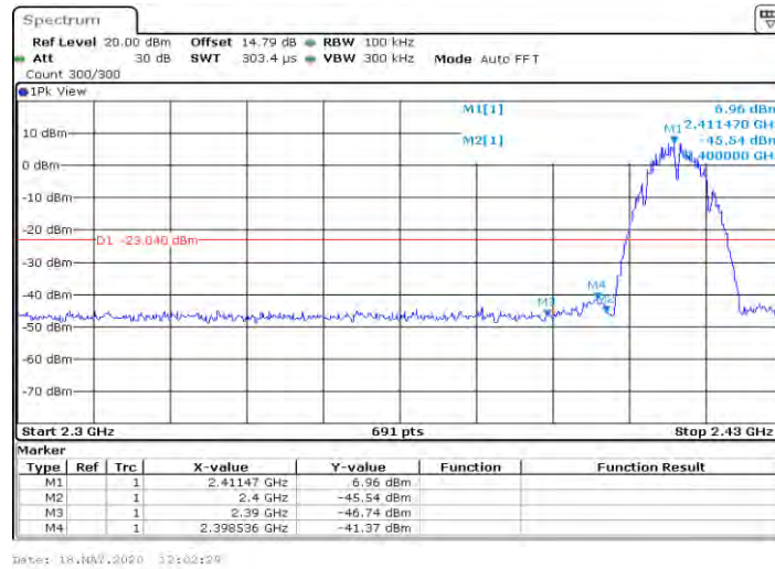
11bMIMO_Ant2_Low_2412
