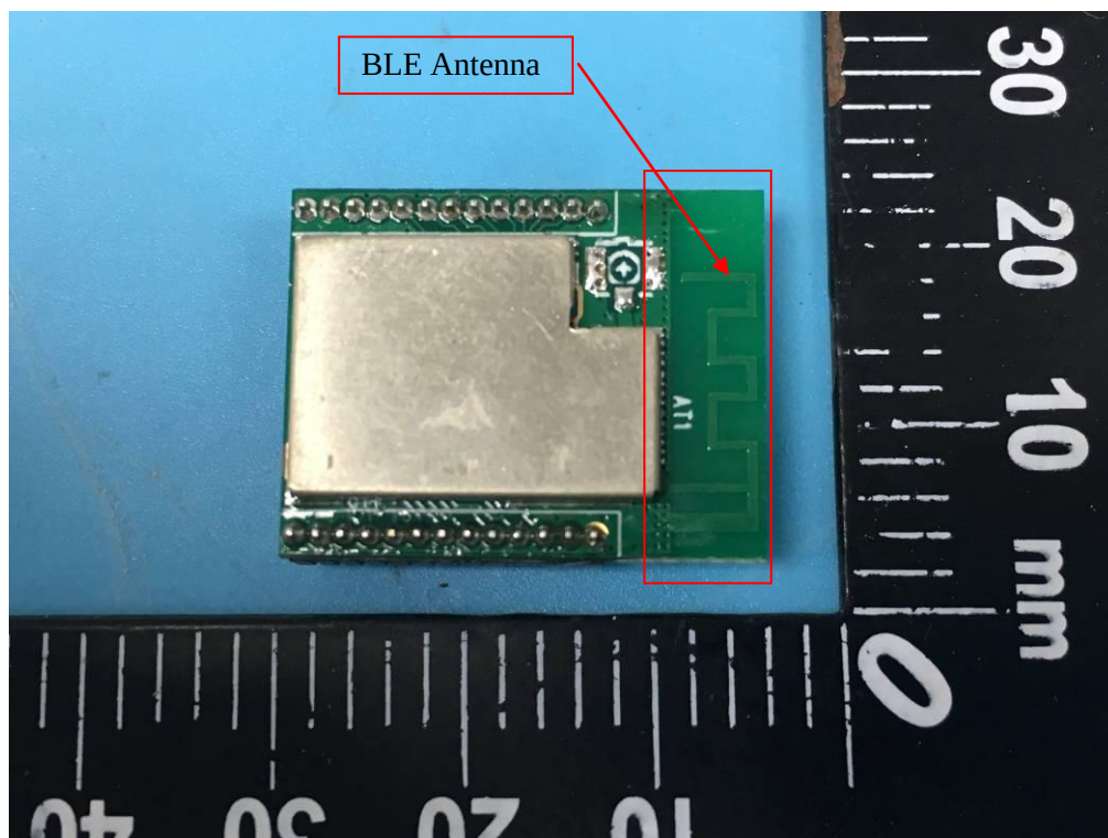
BLE Module
