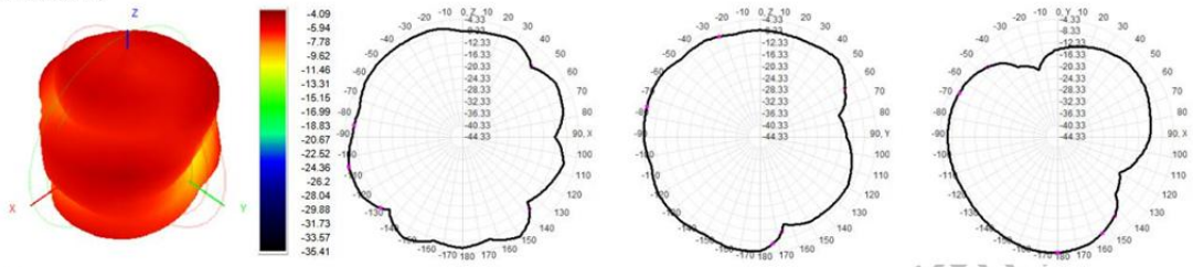
2450MHz
