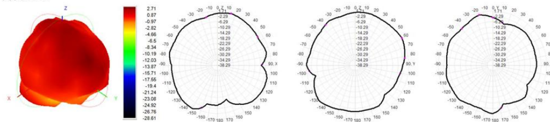
5850MHz
