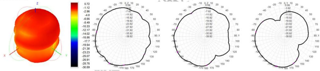
5150MHz
