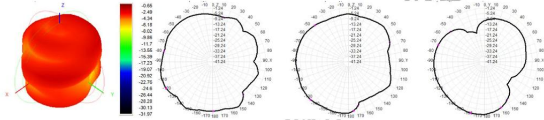
2500MHz
