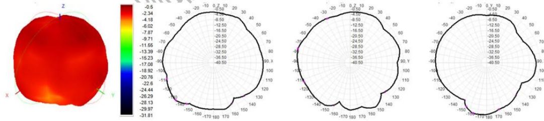
5500MHz
