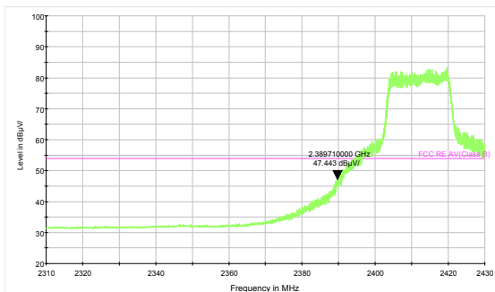
802.11g, Channel No.: 1 - AV
