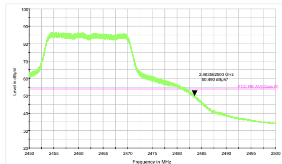
802.11g, Channel No.: 11 - AV
