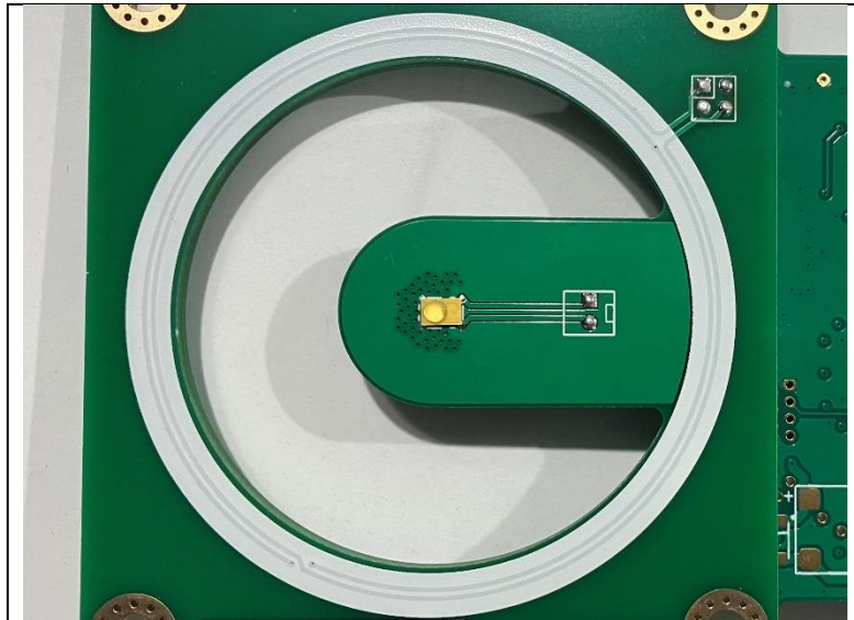
Antenna
