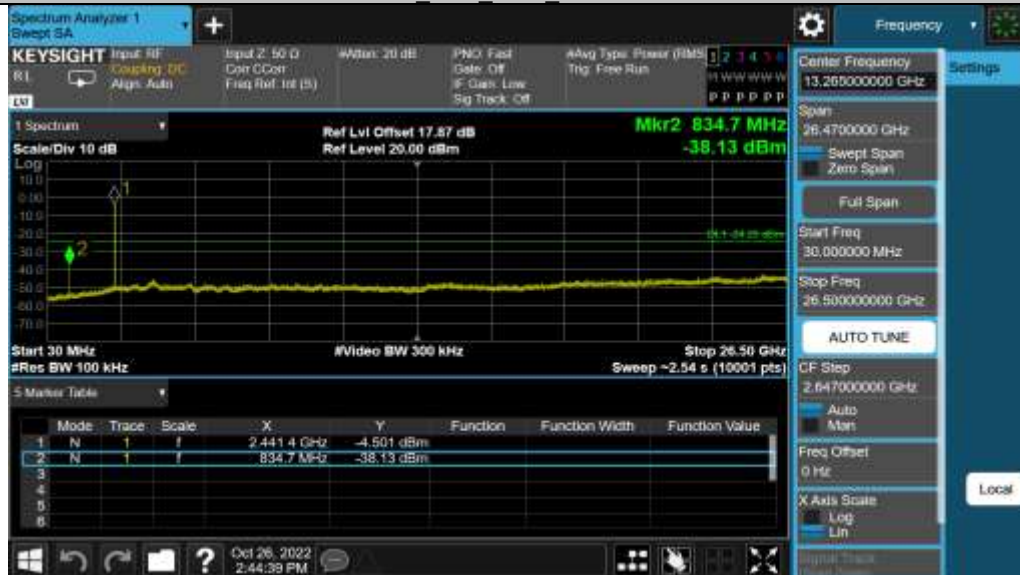
DH5 Ant1 2441 30~26500
