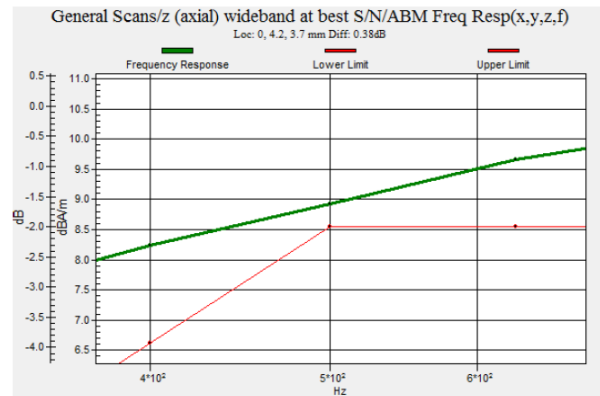
Fig 7.2 GSM850 Ch189
