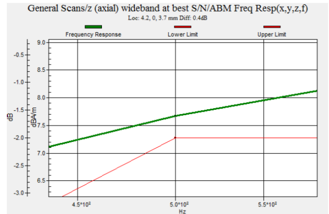
Fig. 7.8 WCDMA Band IV Ch1413
