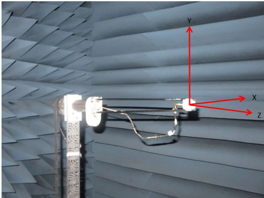
Fig. 4-1 Free Space
