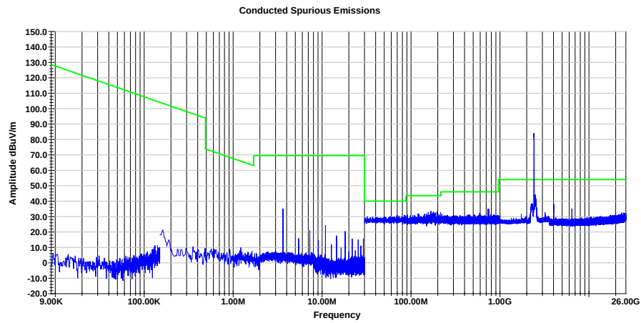
802.11g Ch 1 2412 MHz
