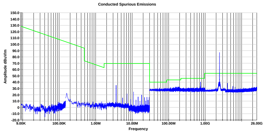
802.11g Ch 13 2472 MHz
