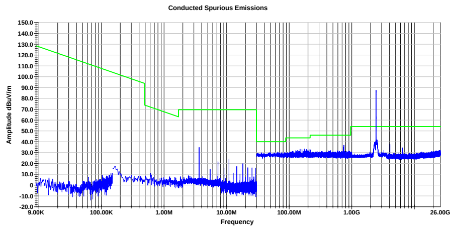
802.11g Ch 7 2442 MHz
