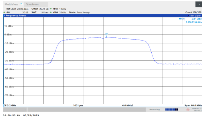
11N20MIMO_Ant2_5200
