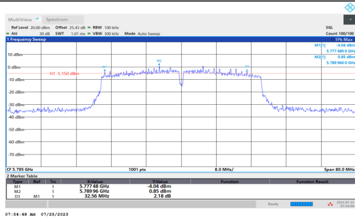
11N40MIMO_Ant2_5795
