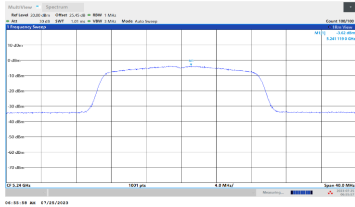
11N20MIMO_Ant2_5240
