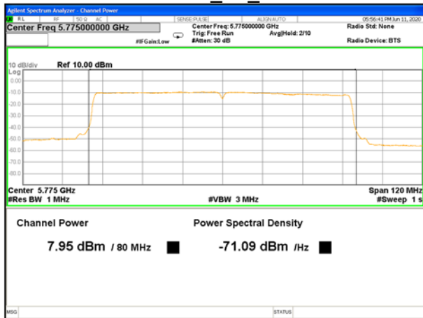
5775MHz_AV_Ant A
