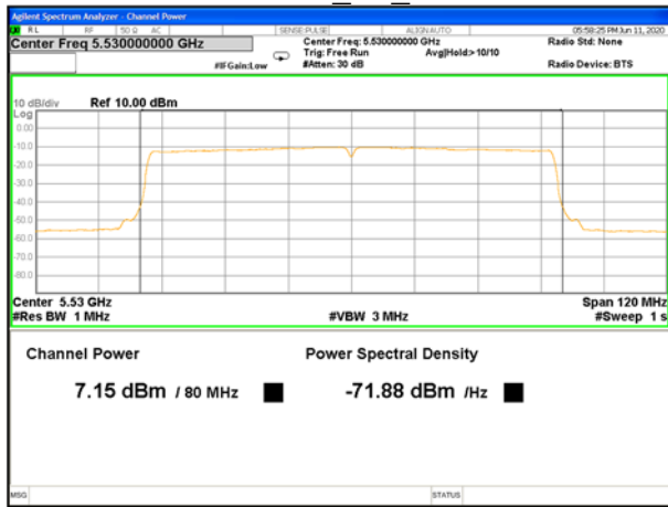
5530MHz_AV_Ant A
