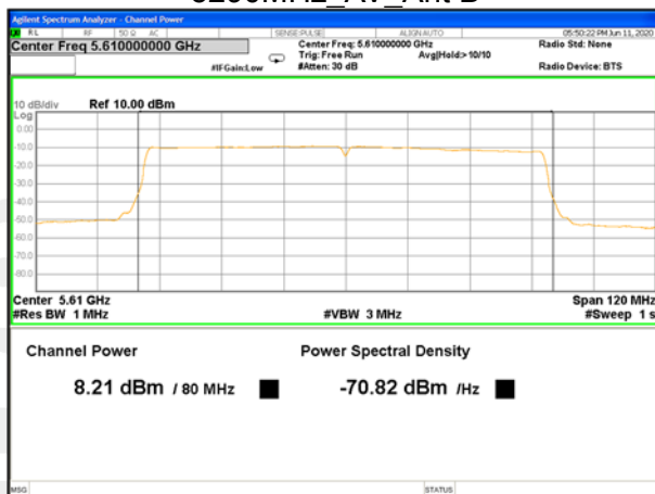
5610MHz_AV_Ant B
