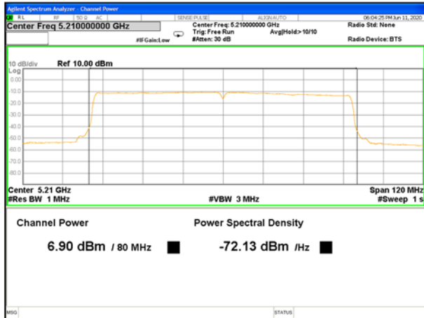
5210MHz_AV_Ant A
