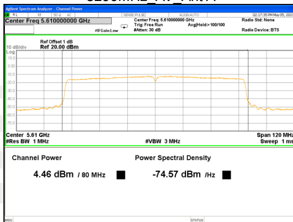
5610MHz_AV_Ant A
