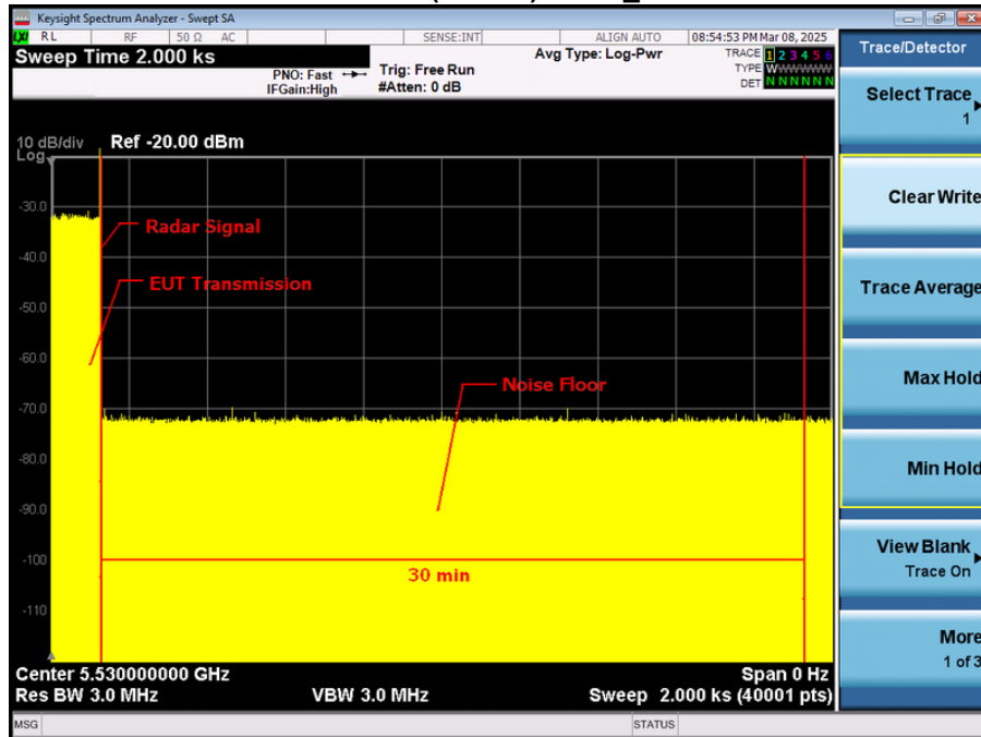
IEEE 802.11ac(VHT80) Mode_5530MHz
