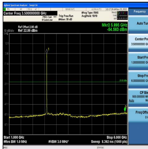
Band41-10MHz-QPSK-40620-50RB#0-Range2:1000~6000MHz
