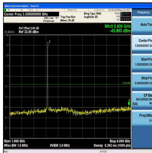
Band7-10MHz-QPSK-21400-50RB#0-Range2:1000~6000MHz
