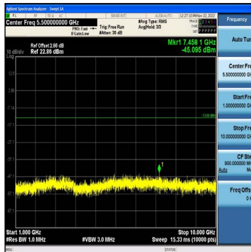
Band5-3MHz-QPSK-20415-15RB#0-Range2:1000~10000MHz
