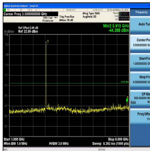
Band7-10MHz-16QAM-21100-50RB#0-Range2:1000~6000MHz
