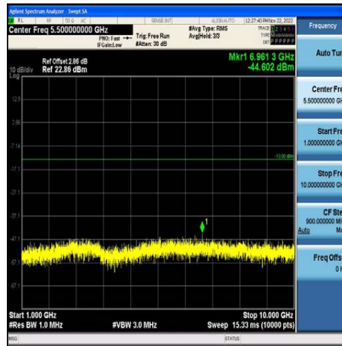
Band5-3MHz-QPSK-20525-15RB#0-Range2:1000~10000MHz
