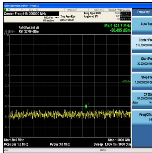
Band7-10MHz-QPSK-21100-50RB#0-Range1:30~1000MHz
