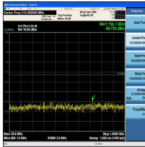
Band4-10MHz-QPSK-20350-50RB#0-Range1:30~1000MHz
