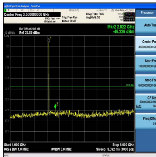
Band7-5MHz-QPSK-21425-25RB#0-Range2:1000~6000MHz
