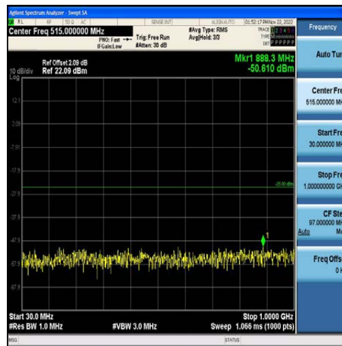
Band7-10MHz-QPSK-21400-50RB#0-Range1:30~1000MHz
