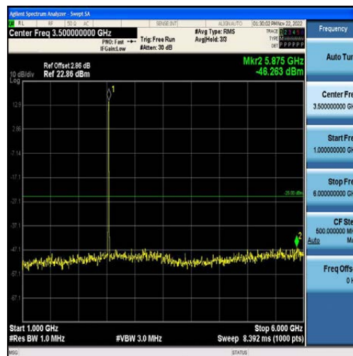
Band7-5MHz-QPSK-21100-25RB#0-Range2:1000~6000MHz
