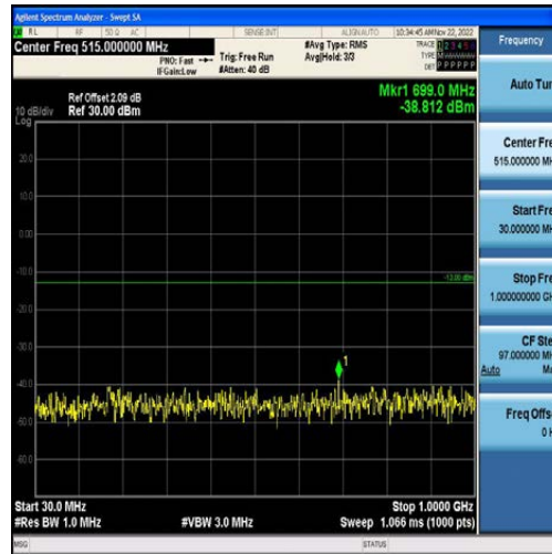
Band4-10MHz-QPSK-20000-50RB#0-Range1:30~1000MHz
