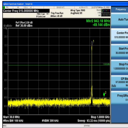
Band5-3MHz-QPSK-20415-15RB#0-Range1:30~1000MHz
