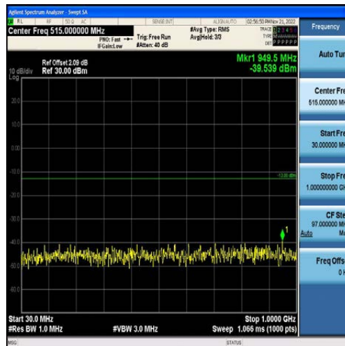
Band2-5MHz-QPSK-18900-25RB#0-Range1:30~1000MHz
