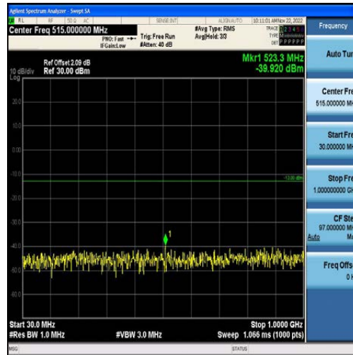
Band4-3MHz-QPSK-19965-15RB#0-Range1:30~1000MHz
