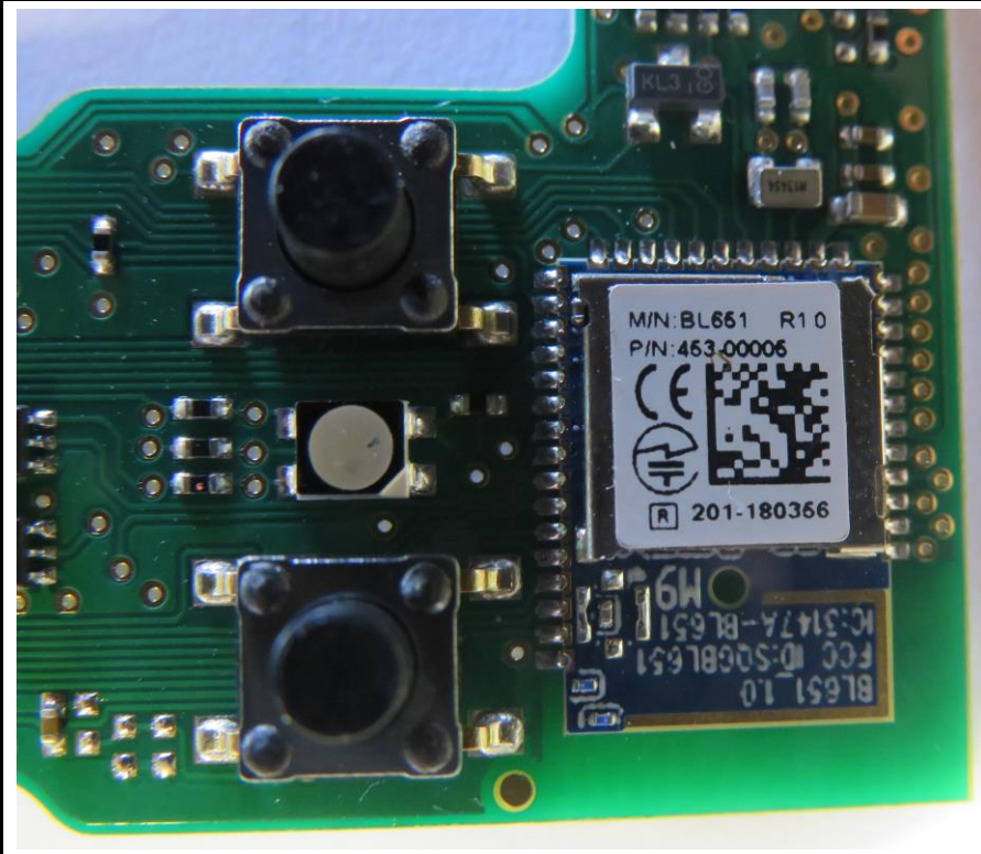
Bluetooth module
