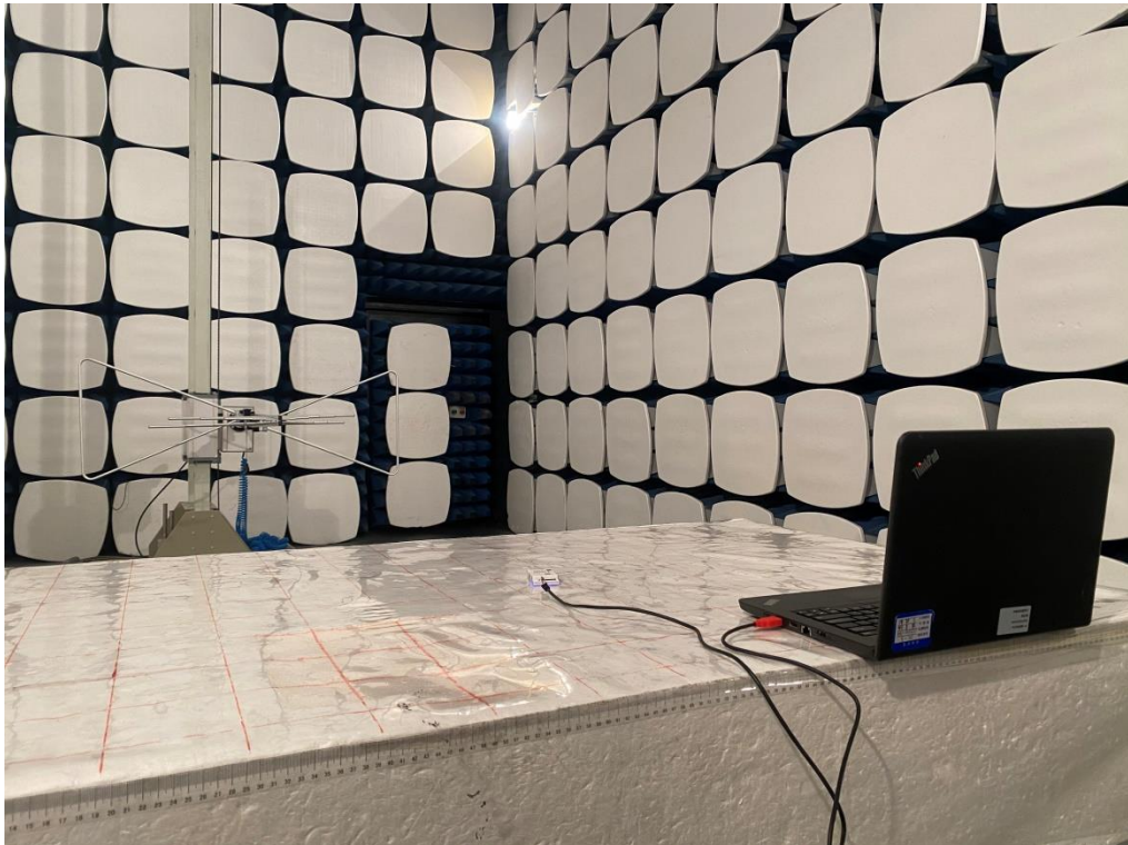
30MHz-1000MHz
