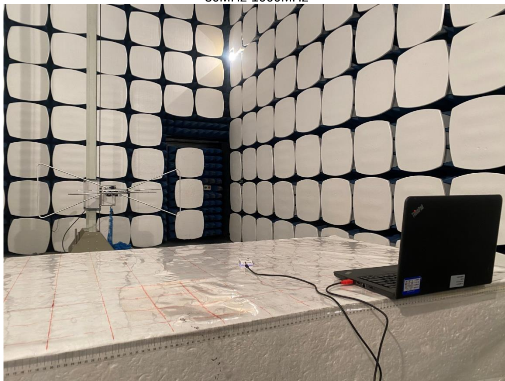
30MHz-1000MHz
