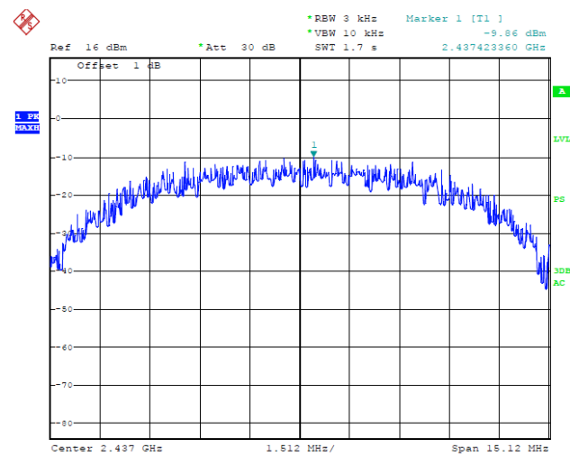
CH6 / 2437 MHz
