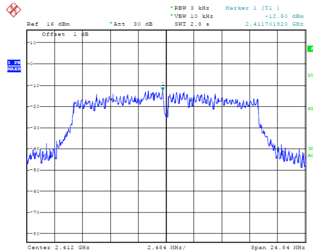
CH1 / 2412 MHz
