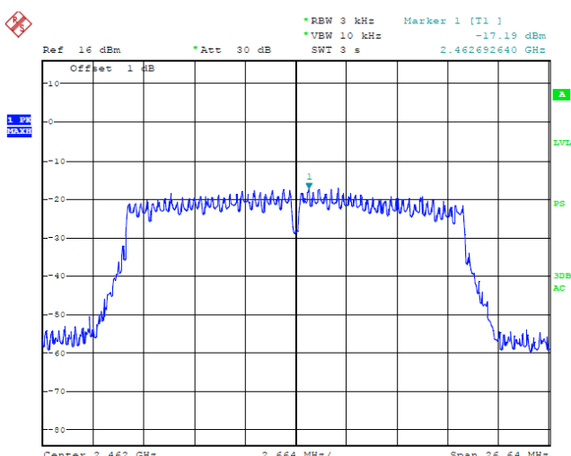
CH11 / 2462 MHz
