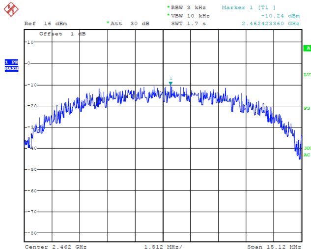
CH11 / 2462 MHz
