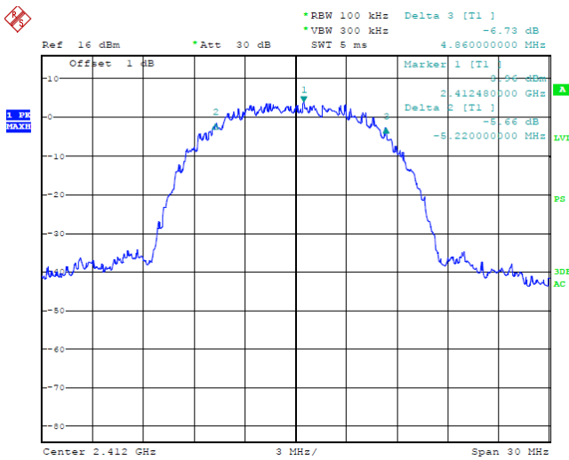
CH1 / 2412 MHz
