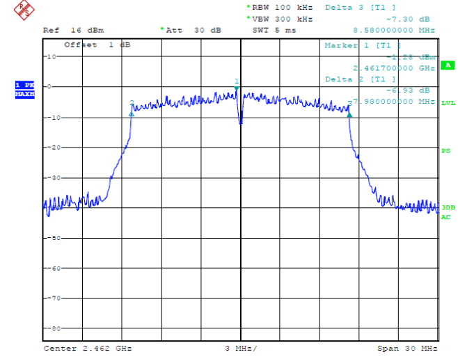
CH11 / 2462 MHz
