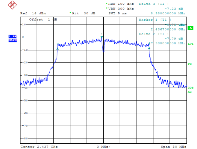
CH6 / 2437 MHz
