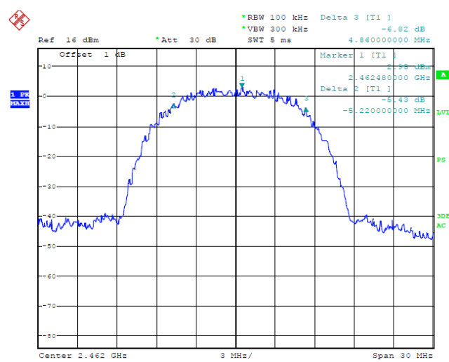
CH11 / 2462 MHz
