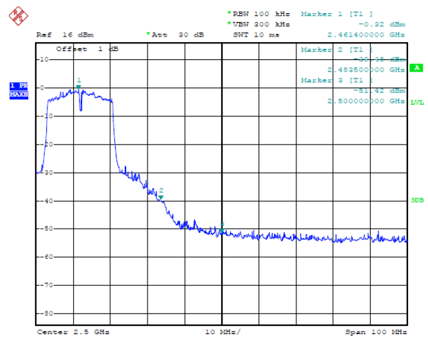
Ch11 / 2462 MHz
