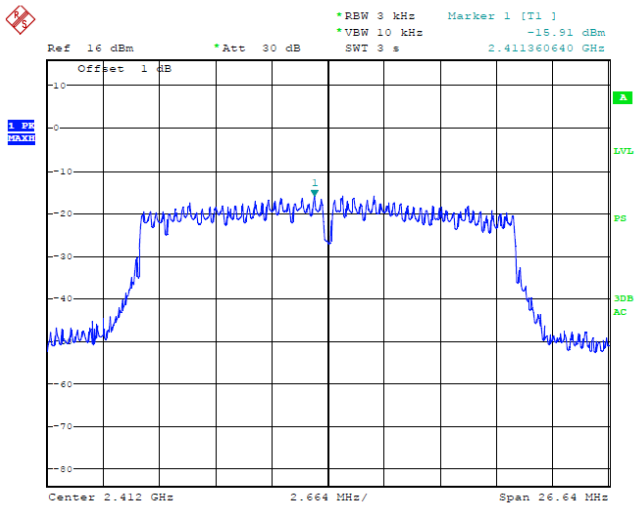
CH1 / 2412 MHz
