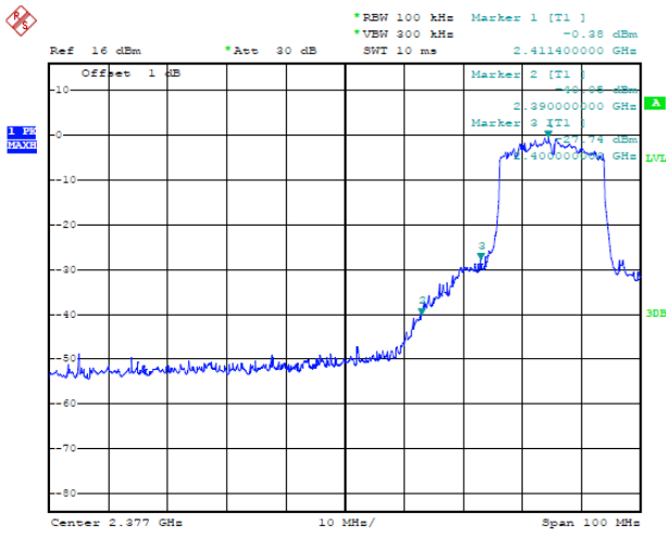
Ch1 / 2412 MHz
