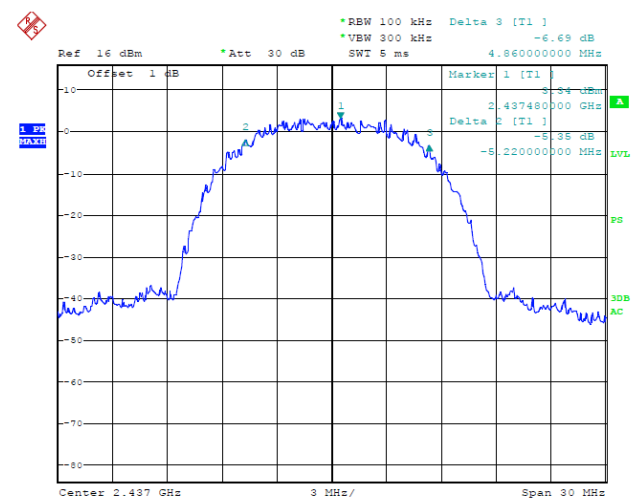
CH6 / 2437 MHz
