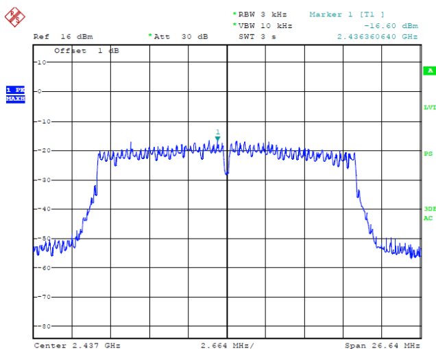
CH6 / 2437 MHz
