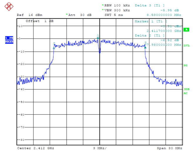
CH1 / 2412 MHz
