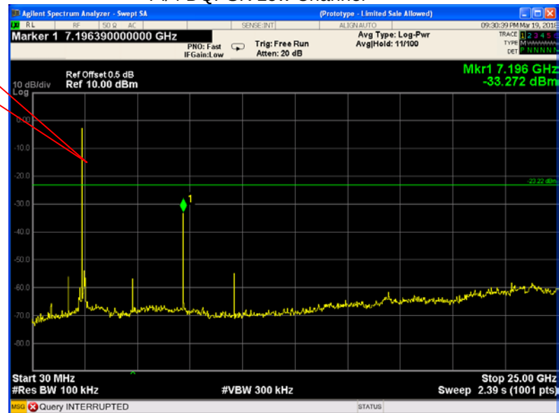
Pi/4 DQPSK Low Channel
