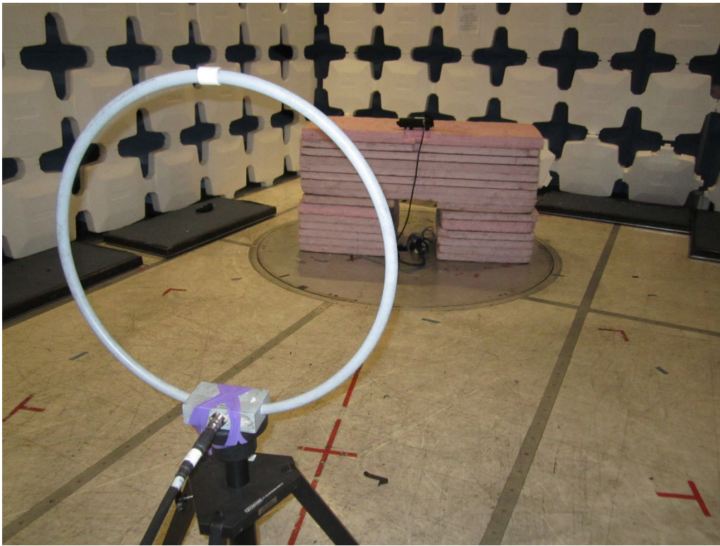
0.150MHz – 1MHz
