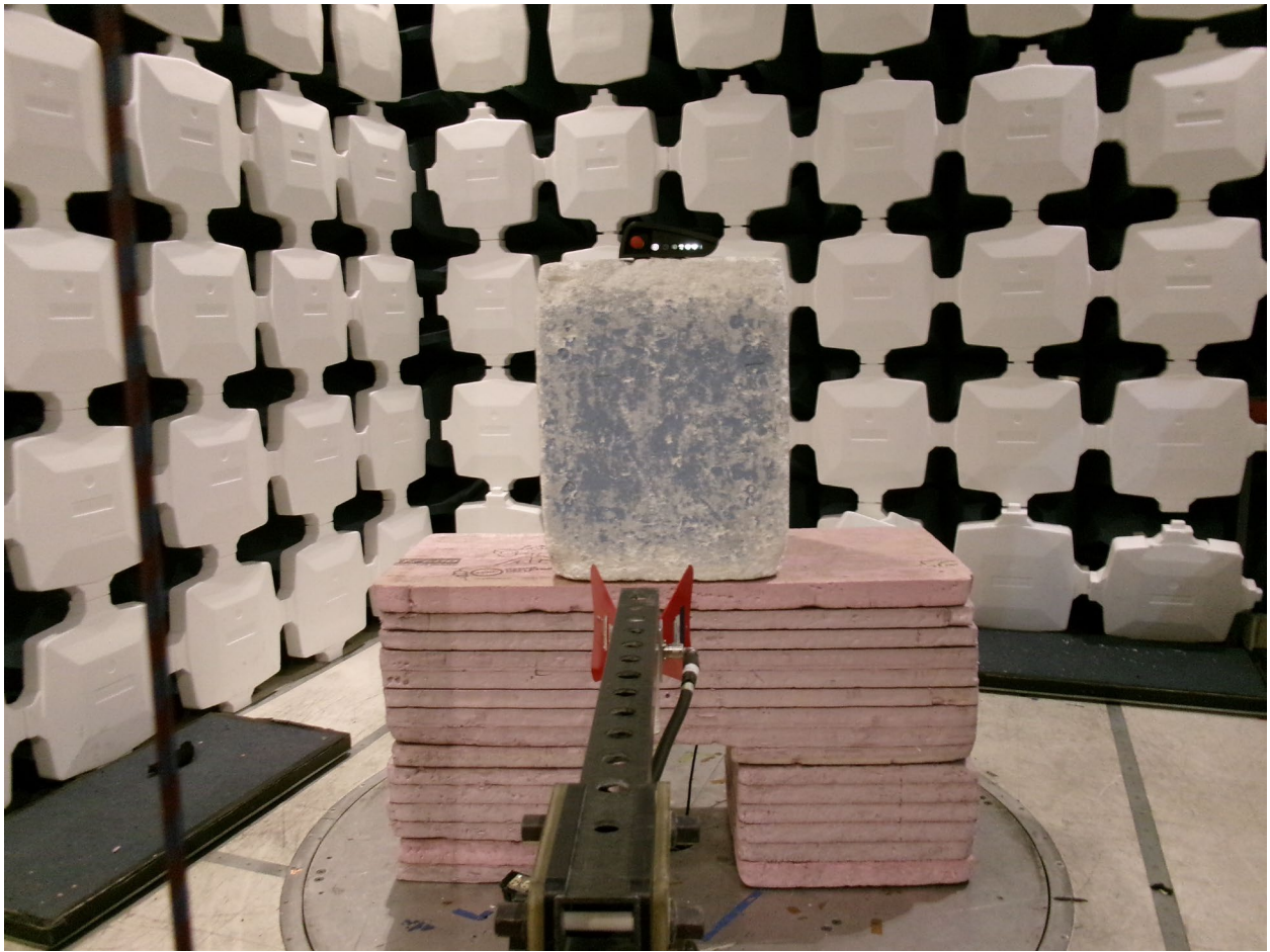
6GHz-10GHz
