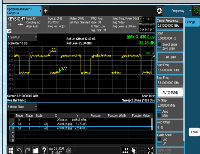
NTNV-11AC80SISO-Ant1-5610
