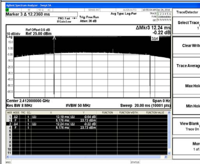
IEEE 802.11b
