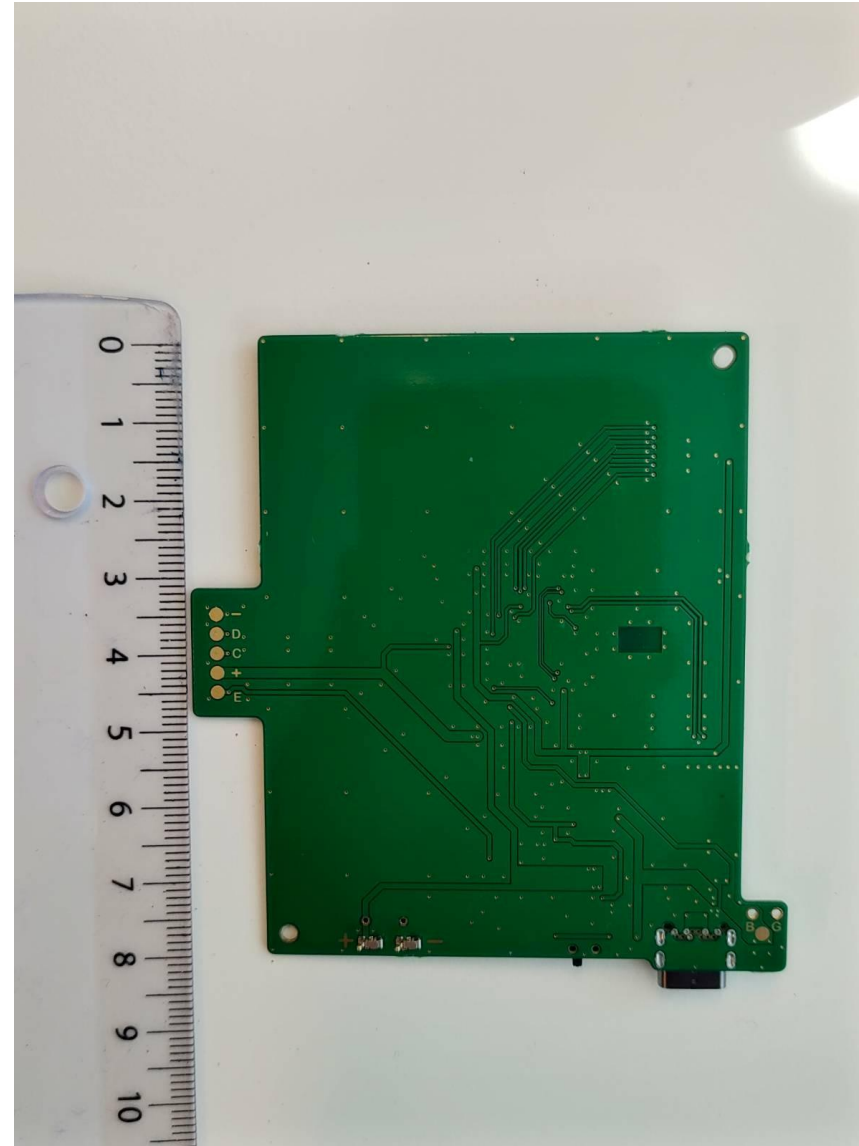
PCB bottom
