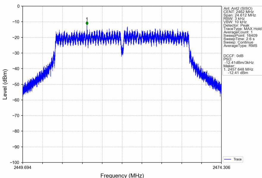
802.11g_HCH_2462MHz_Ant2 (SISO)_NTNV
