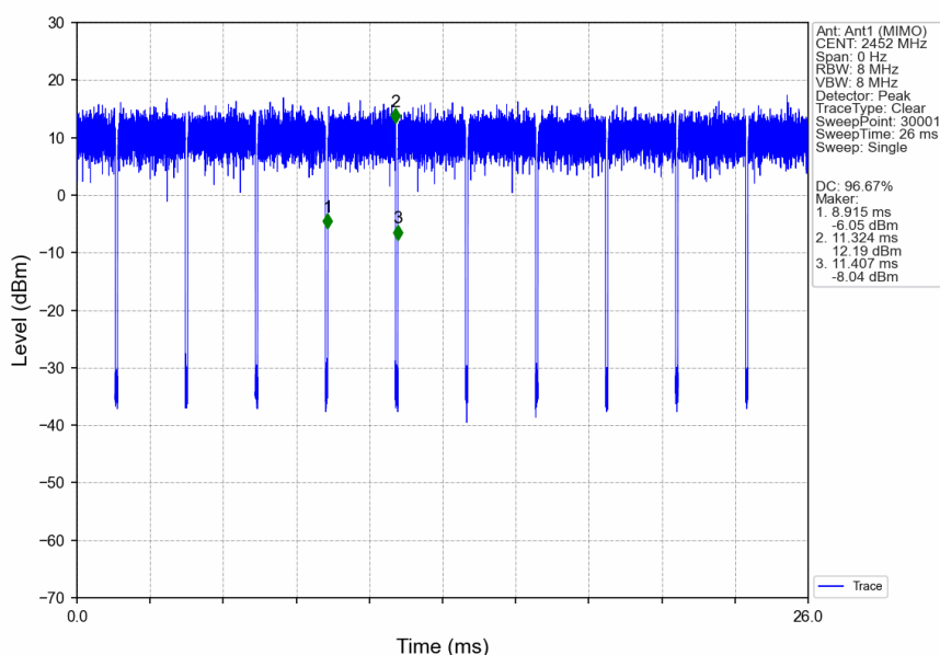
802.11n(HT40)_HCH_2452MHz_Ant1 (MIMO)_NTNV
