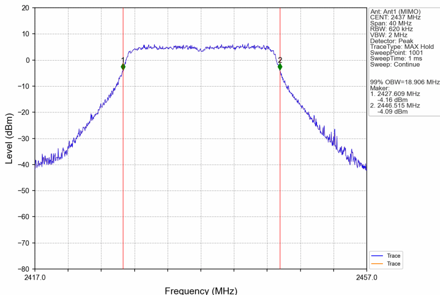
802.11n(HT20)_MCH_2437MHz_Ant1 (MIMO)_NTNV
