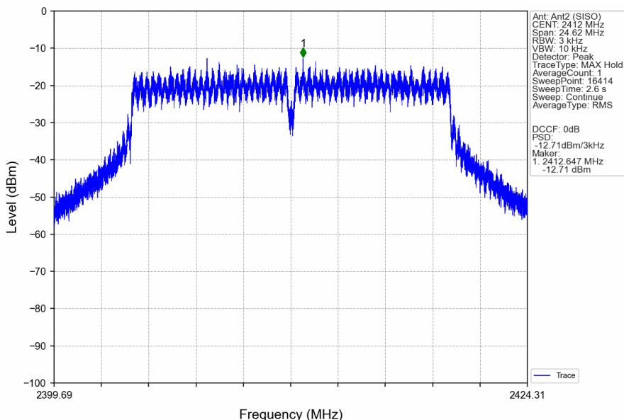
802.11g_LCH_2412MHz_Ant2 (SISO)_NTNV
