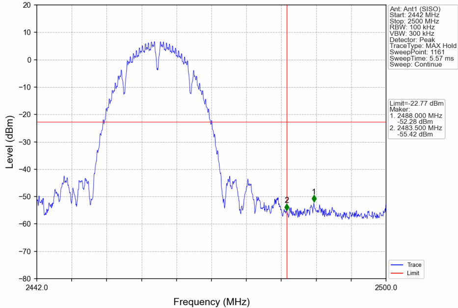
802.11b_HCH_2462MHz_Ant1 (SISO)_NTNV
