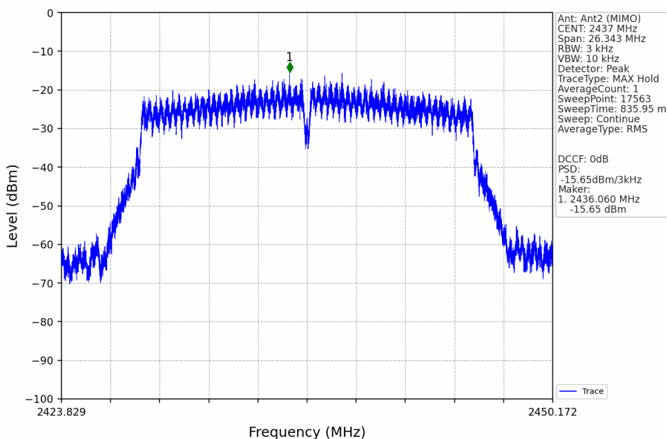
802.11n(HT20)_MCH_2437MHz_MIMO_NTNV
