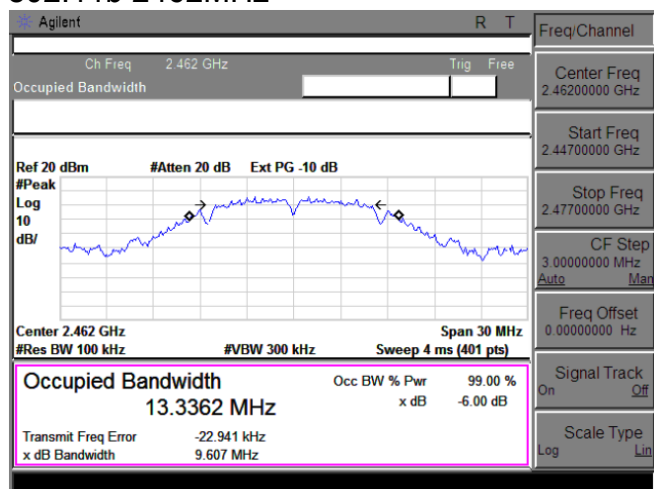
802.11b 2462MHz
