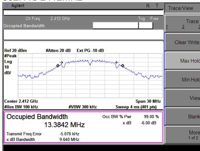
802.11b 2412MHz
