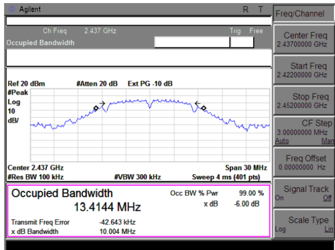
802.11b 2437MHz
