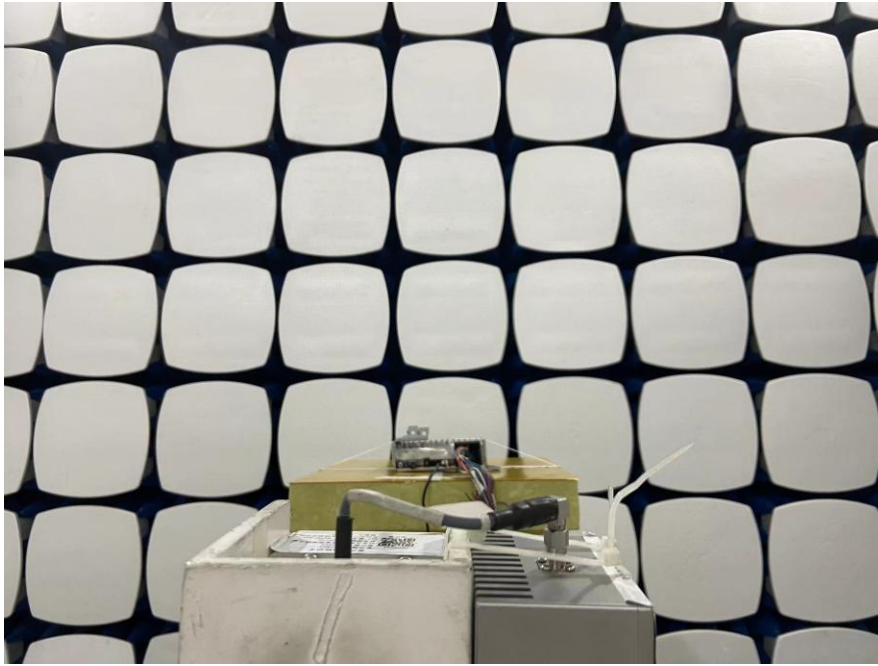
Above 18GHz
