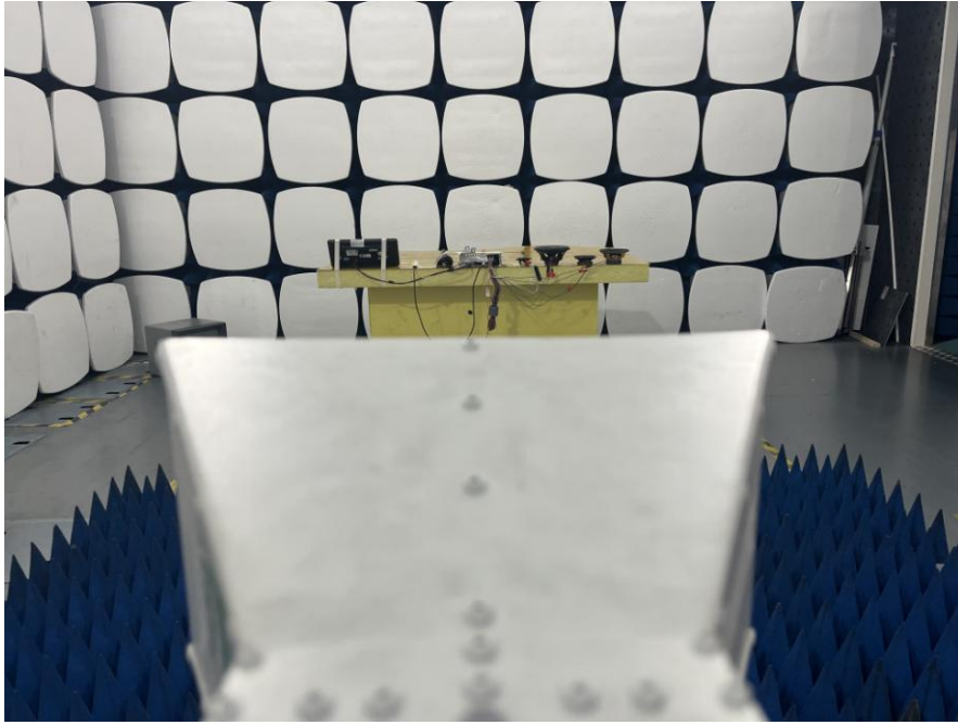
1GHz-18GHz
