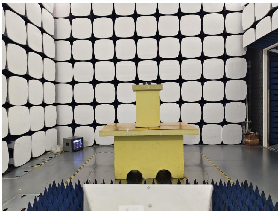
1GHz-18GHz
