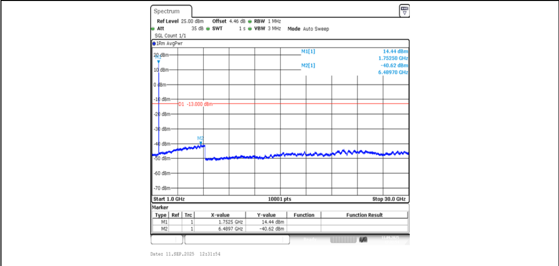
Band4-1513-1000~30000MHz-PASS
