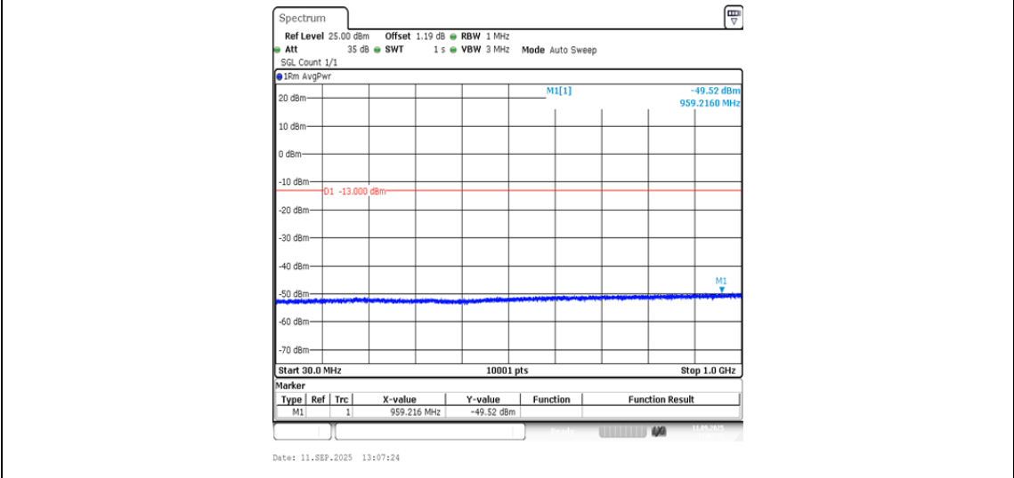
Band4-1312-4-30~1000MHz-PASS
