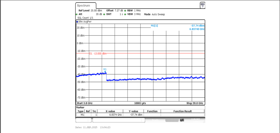
Band4-1312-3-3000~20000MHz-PASS
