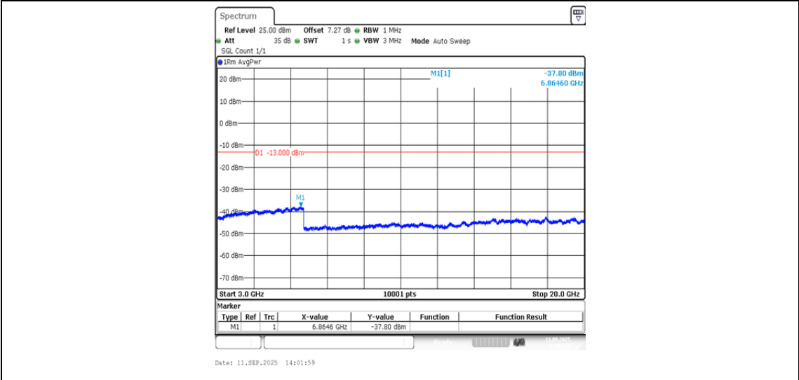
Band4-1312-4-3000~20000MHz-PASS
