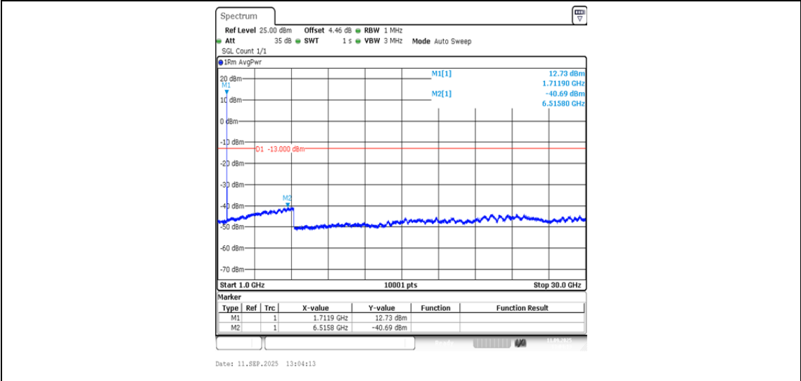
Band4-1312-3-1000~30000MHz-PASS
