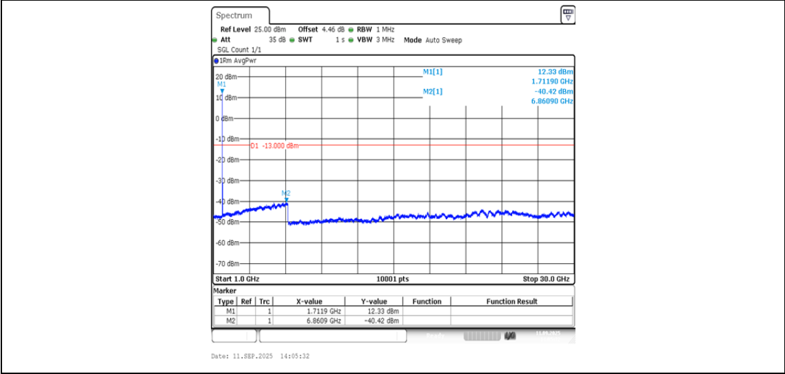
Band4-1312-5-1000~30000MHz-PASS
