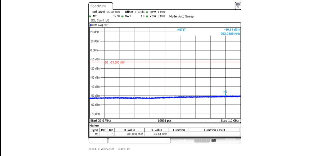
Band4-1312-2-30~1000MHz-PASS
