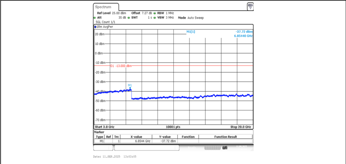
Band4-1513-2-3000~20000MHz-PASS
