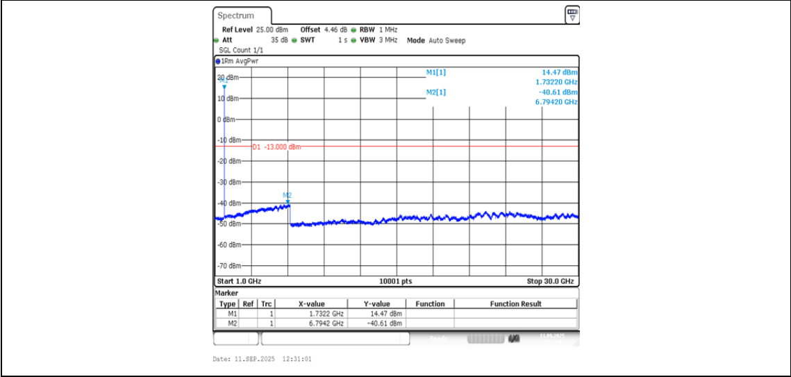
Band4-1413-1000~30000MHz-PASS
