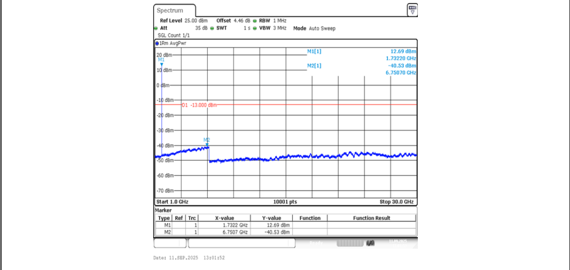
Band4-1413-2-1000~30000MHz-PASS
