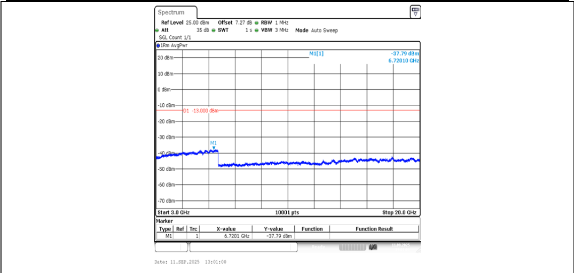
Band4-1312-2-3000~20000MHz-PASS
