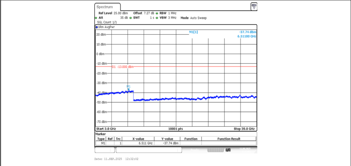
Band4-1513-3000~20000MHz-PASS
