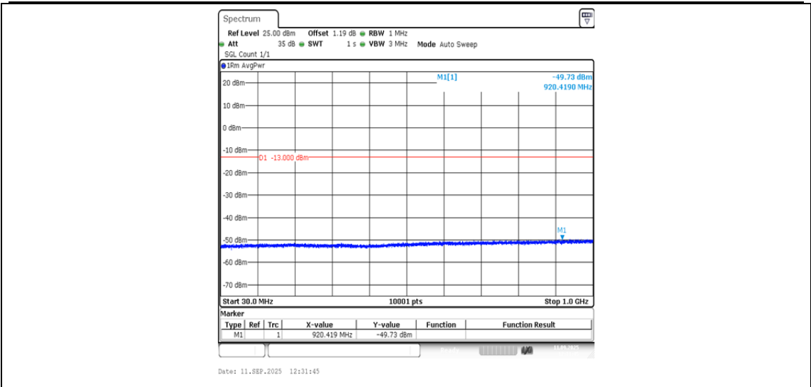
Band4-1513-30~1000MHz-PASS
