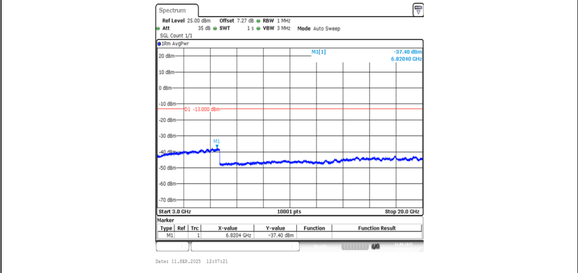
Band2-9400-1-3000~20000MHz-PASS
