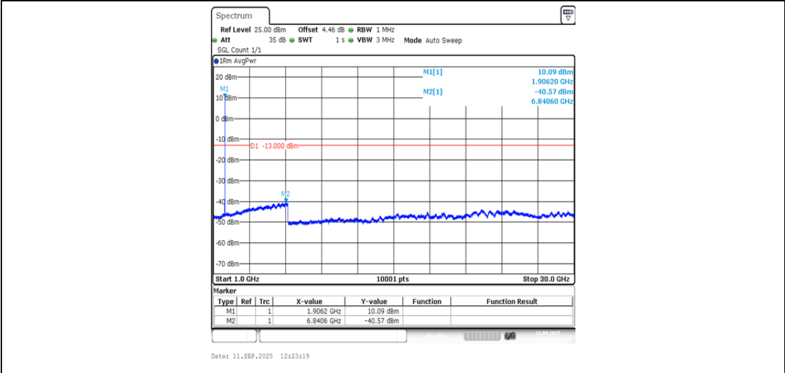
Band2-9538-5-1000~30000MHz-PASS
