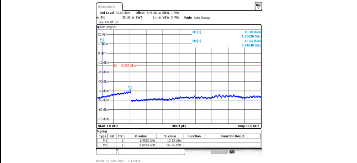
Band2-9538-1-1000~30000MHz-PASS
