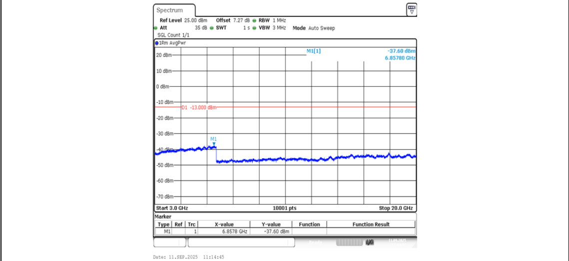
Band2-9538-1-3000~20000MHz-PASS
