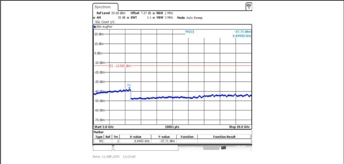
Band2-9262-1-3000~20000MHz-PASS
