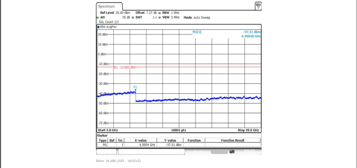
Band4-1513-2-3000~20000MHz-PASS
