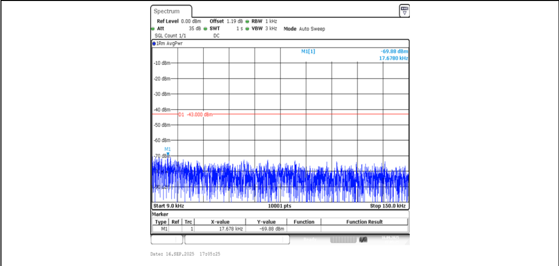
Band4-1513-5-0.009~0.15MHz-PASS
