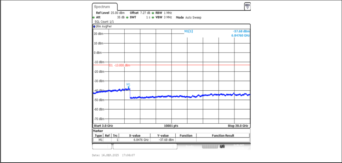
Band4-1513-5-3000~20000MHz-PASS
