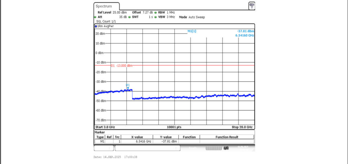
Band4-1413-4-3000~20000MHz-PASS
