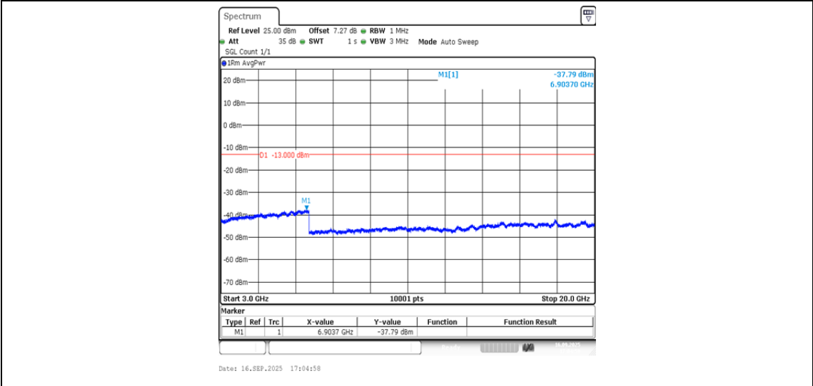
Band4-1413-5-3000~20000MHz-PASS
