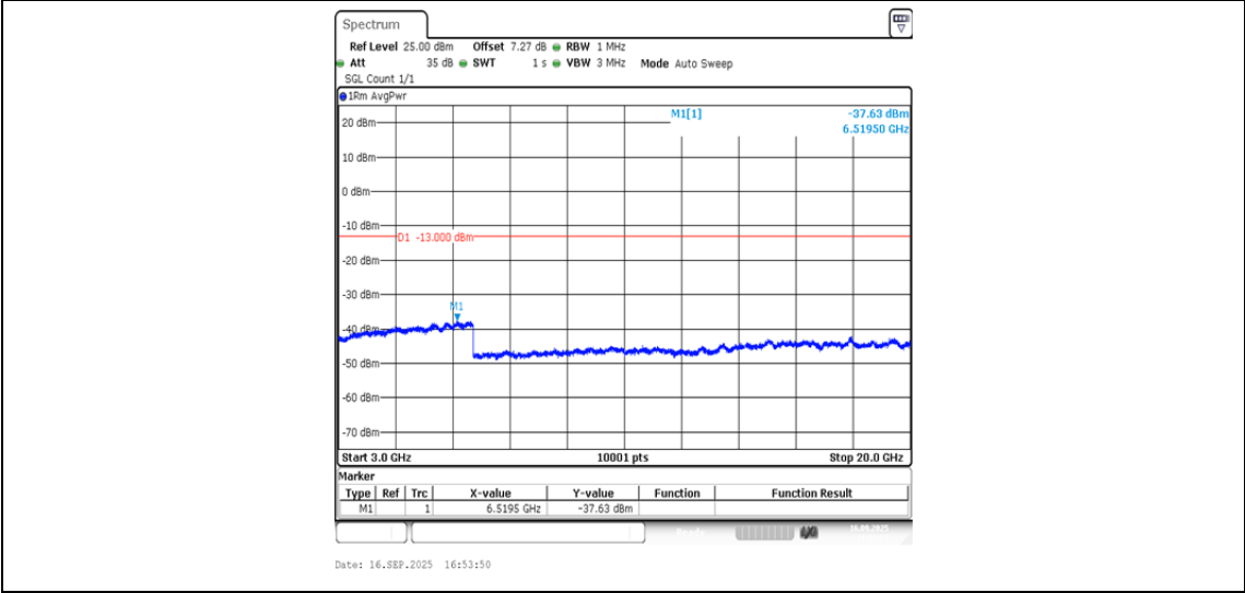
Band4-1312-3-3000~20000MHz-PASS
