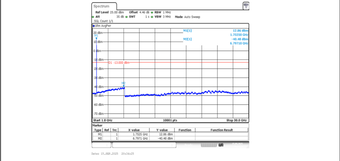
Band4-1513-4-1000~30000MHz-PASS
