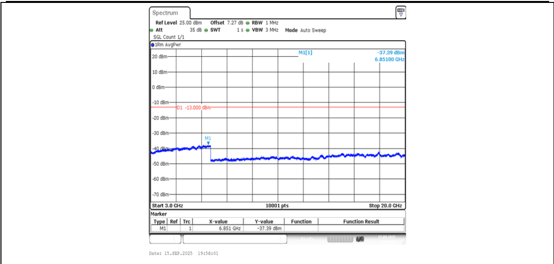
Band4-1413-3000~20000MHz-PASS
