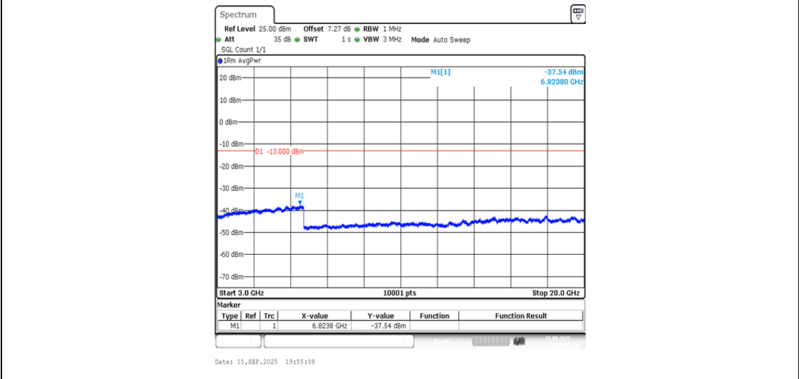
Band4-1312-3000~20000MHz-PASS
