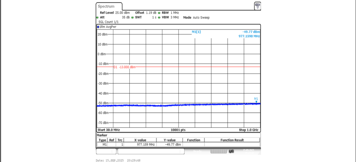
Band4-1413-3-30~1000MHz-PASS
