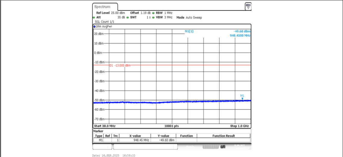
Band4-1312-4-30~1000MHz-PASS
