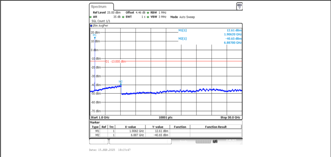
Band2-9538-1-1000~30000MHz-PASS
