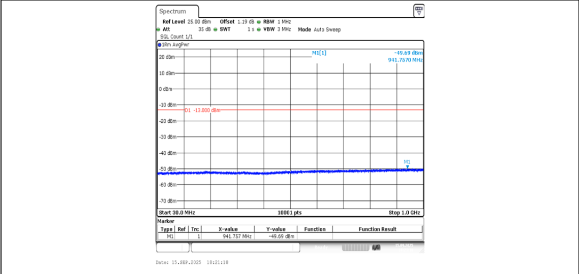
Band2-9400-3-30~1000MHz-PASS
