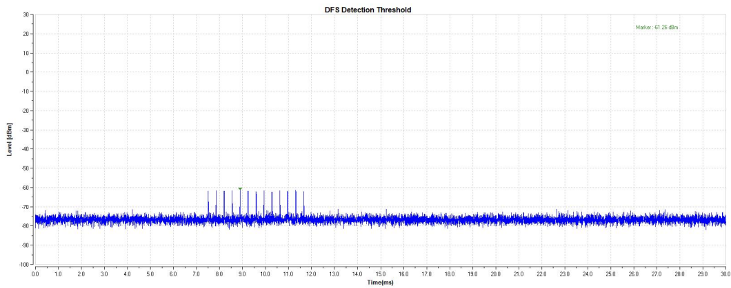
11AC80SISO-5290-Type4-PASS
