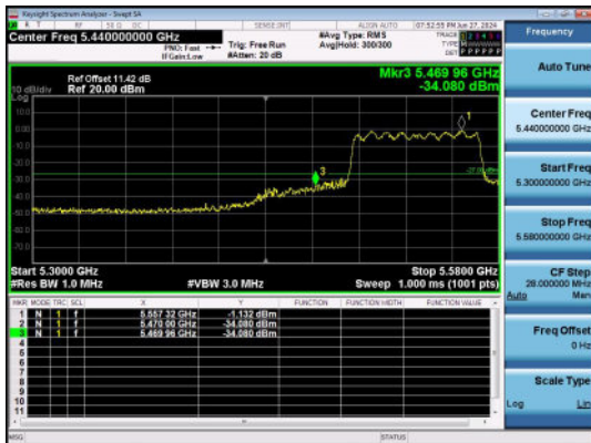
11AC80SISO-Ant1-5530-PASS
