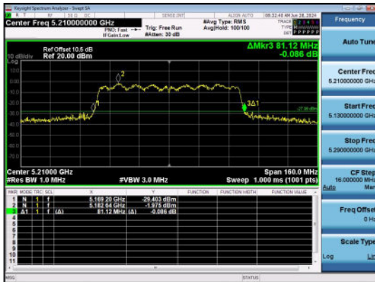
11AC80SISO-Ant1-5210-26dB EBW
