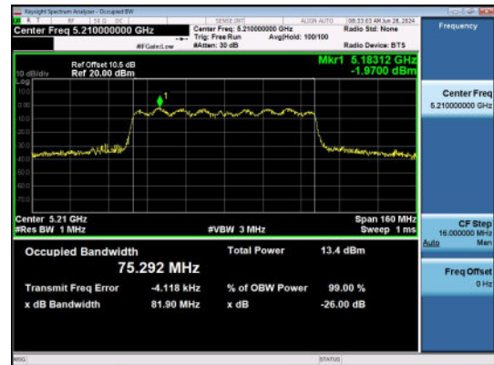
11AC80SISO-Ant1-5210-99% OBW
