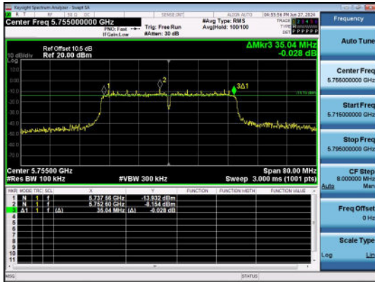
11N40SISO-Ant1-5755-PASS
