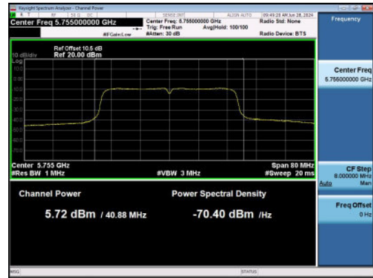
11N40SISO-Ant1-5755-PASS
