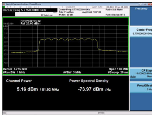
11AC80SISO-Ant1-5775-PASS
