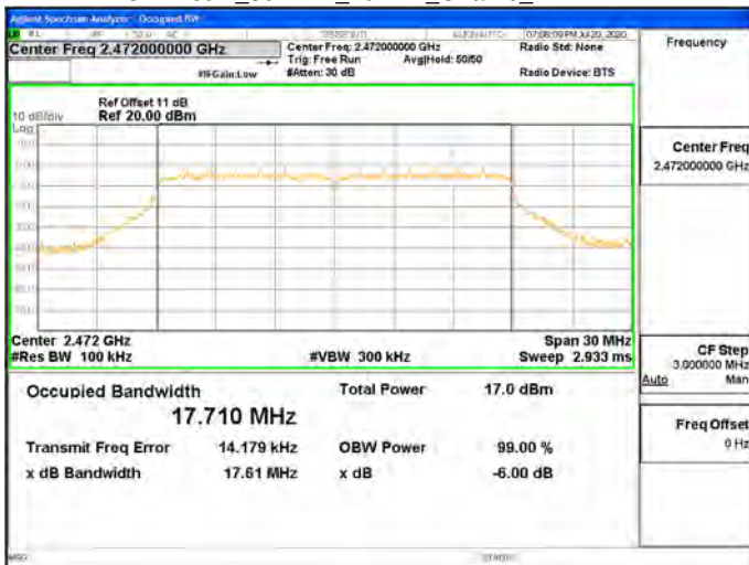
OBW 6dB_802.11n_20MHz_Chain0_2472MHz
