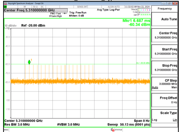
HE40_5310MHz_Type 1-A
