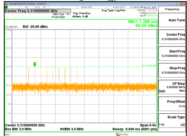
HE40_5310MHz_ype 6
