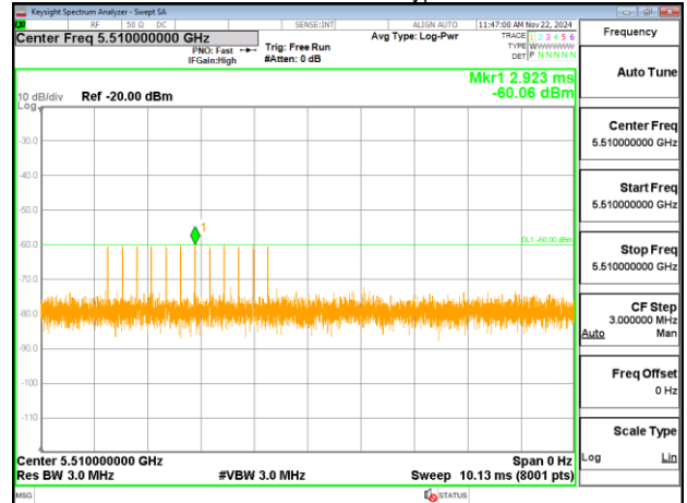
HE40_5510MHz_Type 4
