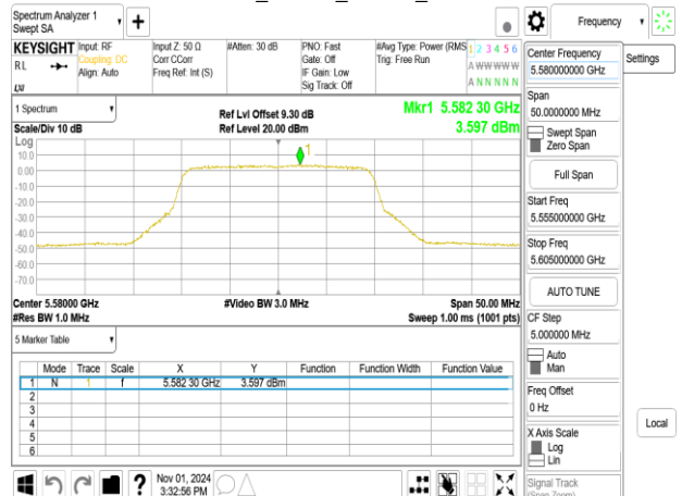
802.11ax_20MHz_Chain1_5580MHz
