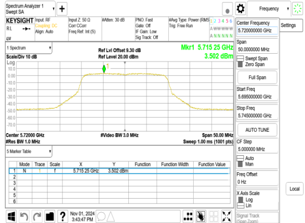
802.11ax_20MHz_Chain0_5720MHz_UNII 2C
