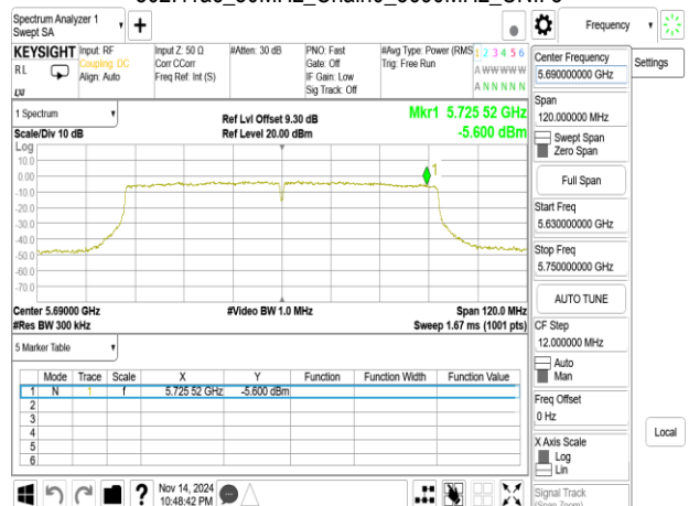
802.11ac_80MHz_Chain0_5690MHz_UNII 3
