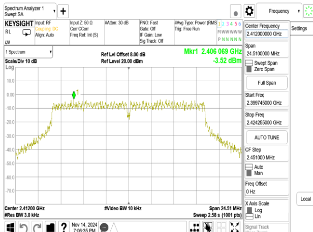
802.11g_20MHz_Chain1_2412MHz
