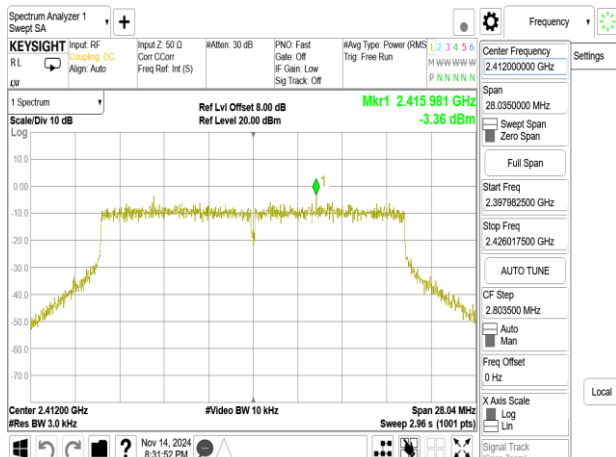
802.11ax_20MHz_Chain1_2412MHz
