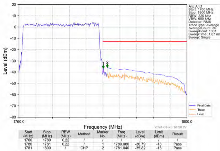
Band66 20MHz 16QAM HCH 1770MHz RB 100 0 NTNV
